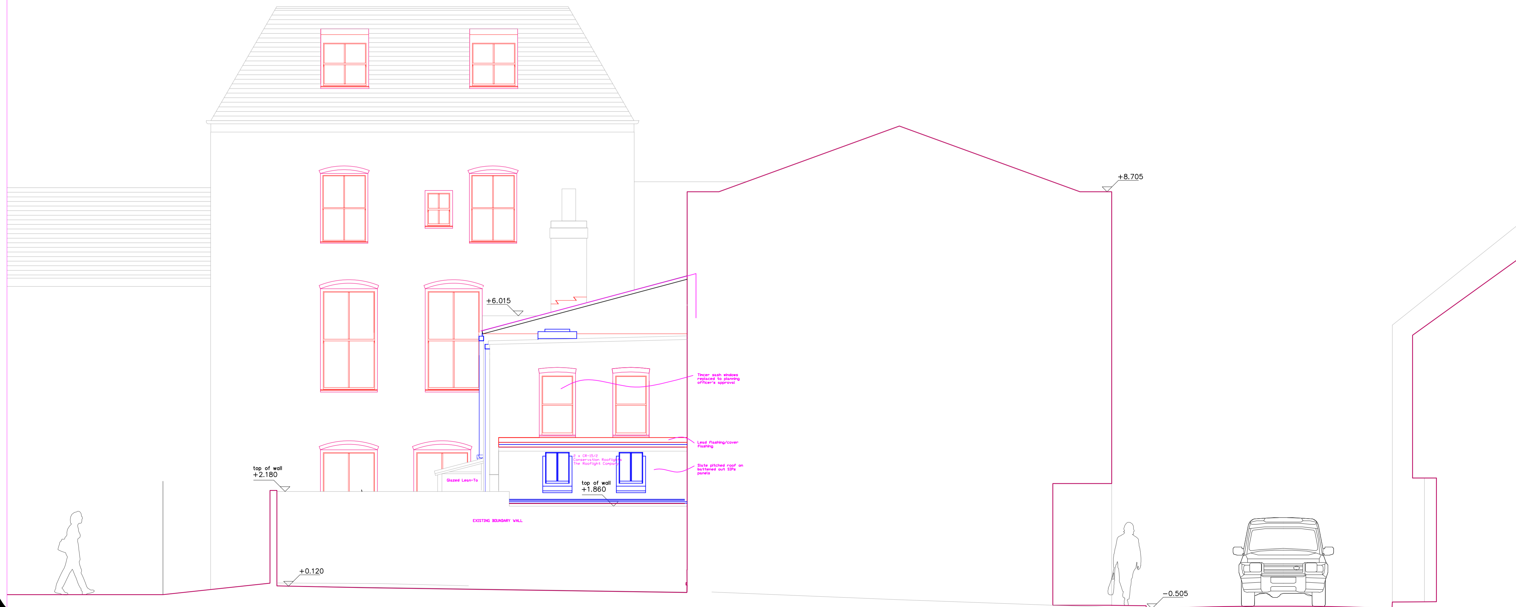
SECTION DD
